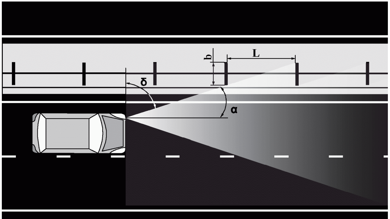
Рисунок 3. Определение угла падения светового потока ( \alpha ) ограничивающего угла ( \delta ): b - ширина затемняющего элемента; L - расстояние между затемняющими элементами
